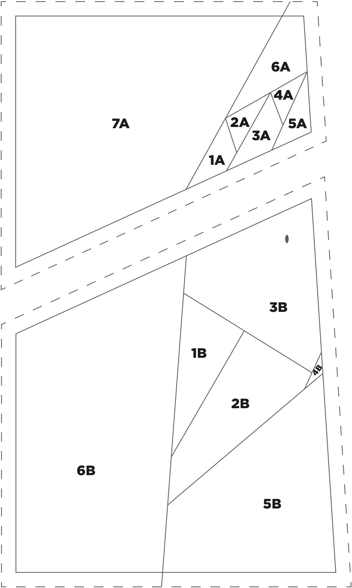
PRETTY POLLY Cockatoo Section A ACTUAL SIZE
